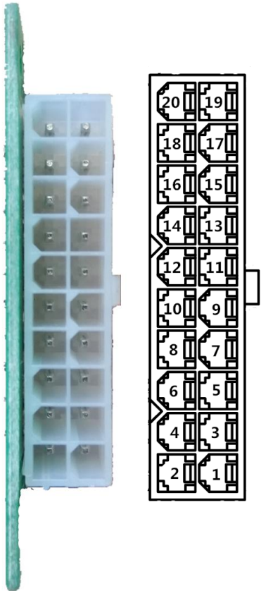
图 2.2 J5 端子序号图
