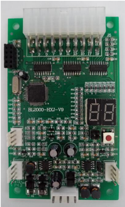
图 2.1 BL2000-HXJ-V9 实物图
