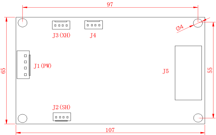
图 2.3 BL2000-HXJ-V9 尺寸图（单位 mm）
